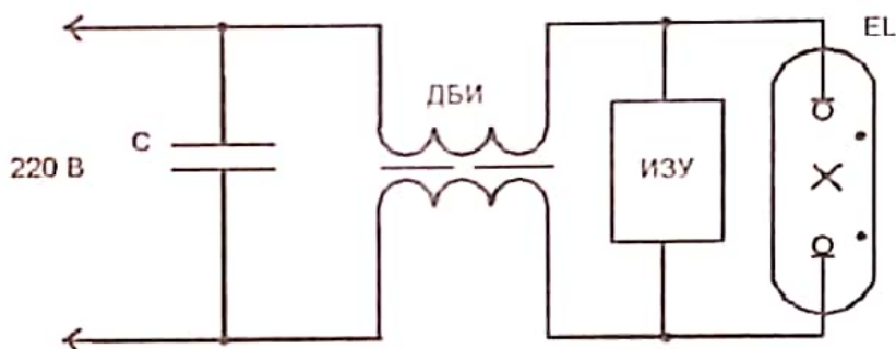
Рисунок 4. Схема включения ламп ДРИ: С - конденсатор; EL - лампа ДРИ; ДБИ – дроссель балластный индуктивный, ИЗУ – импульсное зажигающее устройство.
