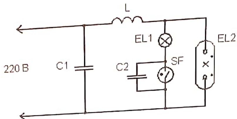
Рисунок 5. Схема відключення ламп ДНаТ: C1 и C2 - конденсаторы; EL1 - лампа накаливания; EL2 - лампа ДНаТ; L - дроссель, SF - стартер.
