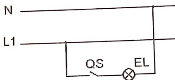
Рисунок 1. Схема включения электрических ламп накаливания
