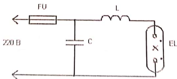
Рисунок 3. Схема включения лампы ДРЛ: FU - предохранитель; C - конденсатор; EL - лампа ДРЛ; LL - дроссель.
