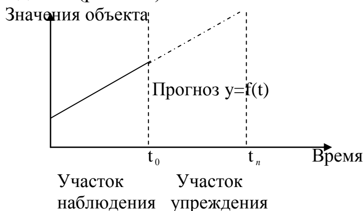
Рис. 2.1. Экстраполяция тренда
