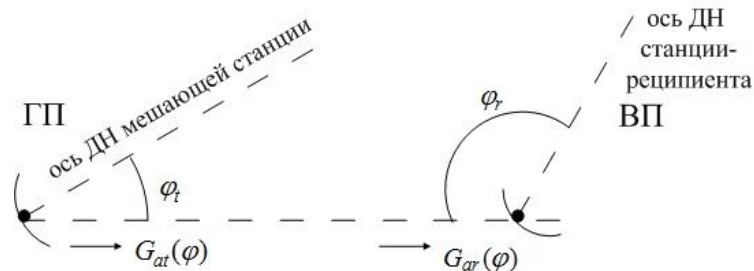
Рисунок 1 – Помеховая ситуация в тракте магистральной связи
