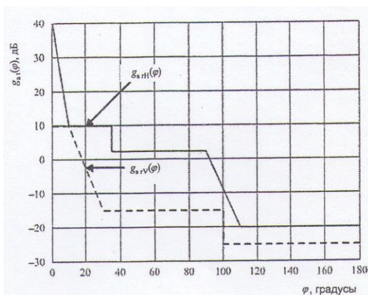
Рисунок 2 – Пример зависимости коэффициента усиления передающей антенны мешающей станции для основной и кроссполаризации
