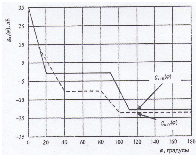
Рисунок 3 – Пример зависимости коэффициента усиления приемной антенны станции-реципиента для основной и кроссполаризации
