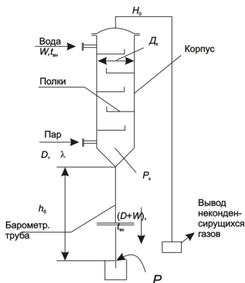
Рис. 4.4. Принципиальная схема конденсатора смешения с барометрической трубой
