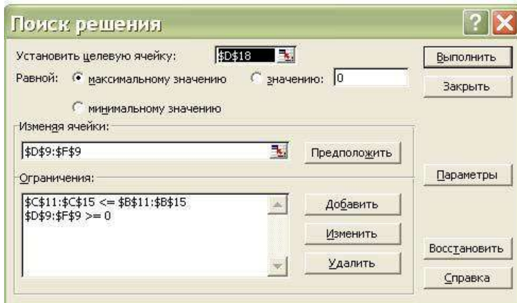
Рис. 3. Пример заполнения окна «Поиск решения»
