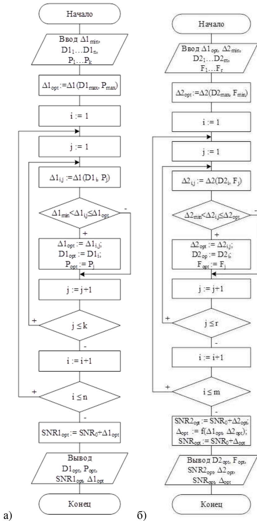
Рисунок 1 – Алгоритмы оптимизации параметров земных станций: а) 3C_1 ; б) 3C_2
